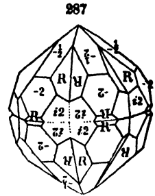
Chabazite.
